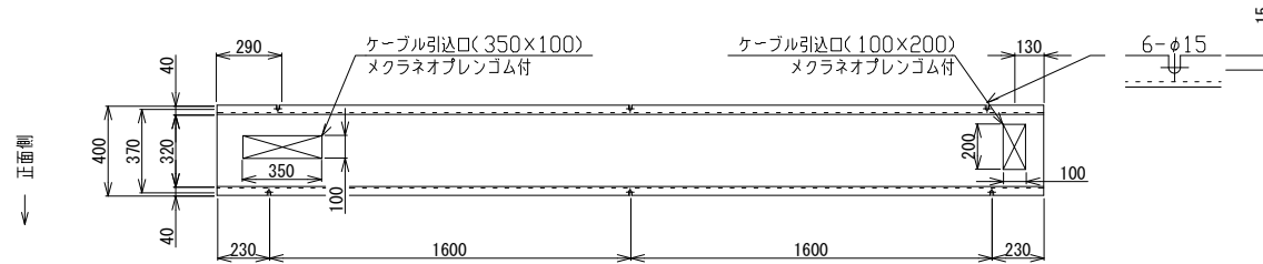
(ケース上面から見たベース詳細図)
