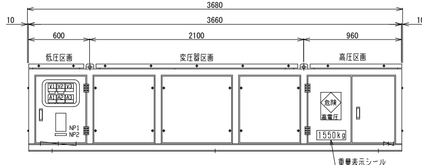
正面図
