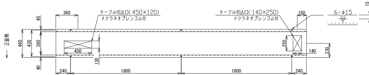
(ケース上面から見たベース詳細図)
