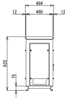
左側面図
