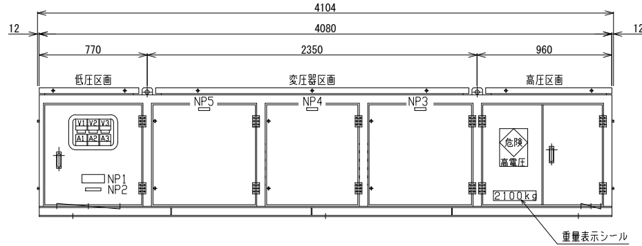
正面図
