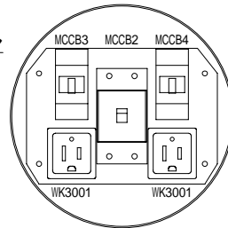
2次側パネル
