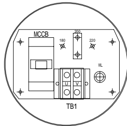
1次側パネル
